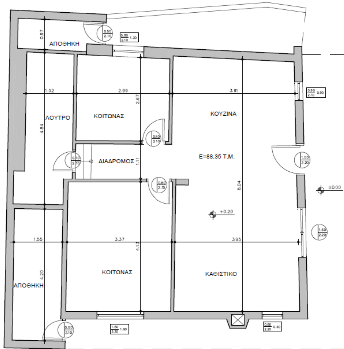
ΚΑΤΟΨΗ ΙΣΟΓΕΙΑΣ ΚΑΤΟΙΚΙΑΣ
